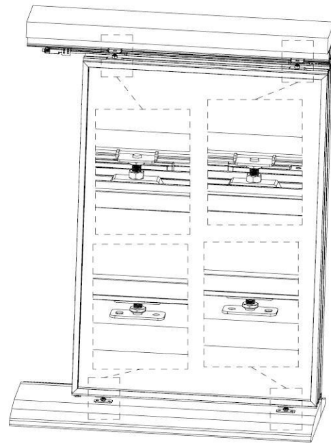
10、安装固定门
